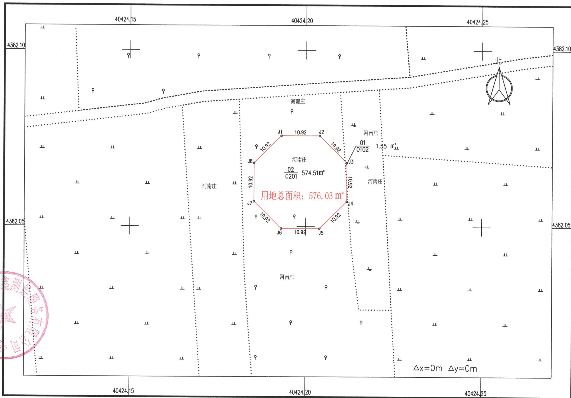
金风昌黎县 200MW 风力发电项目 (7号机位) 建设用地勘测定界图
