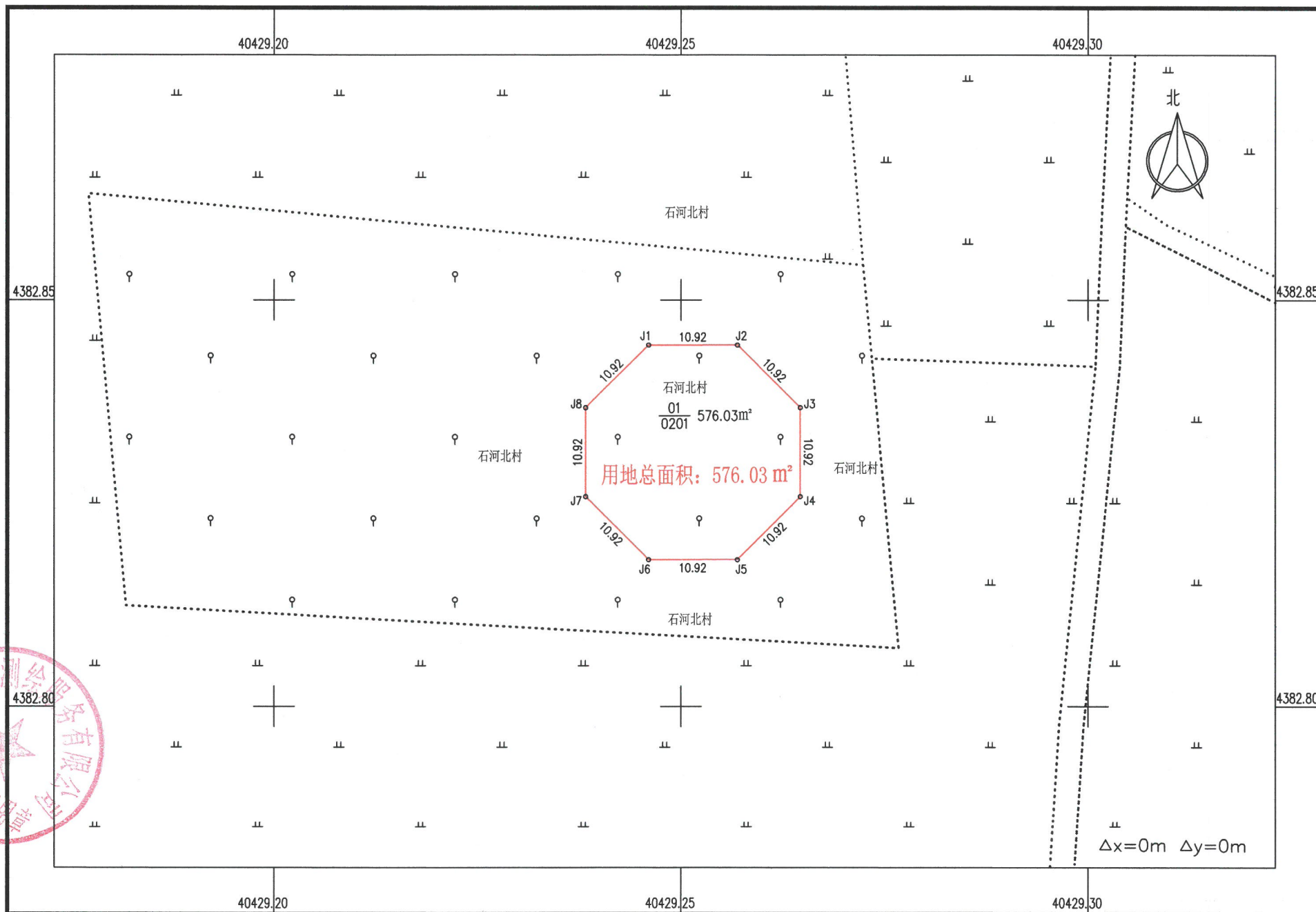
金风昌黎县 200MW 风力发电项目 (22号机位) 建设用地勘测定界图
