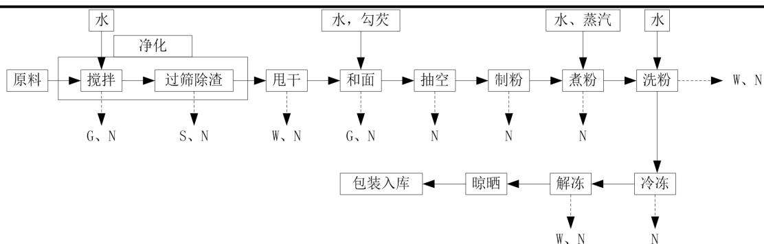
图2-2 现有工程一号、三号生产线工艺流程图
