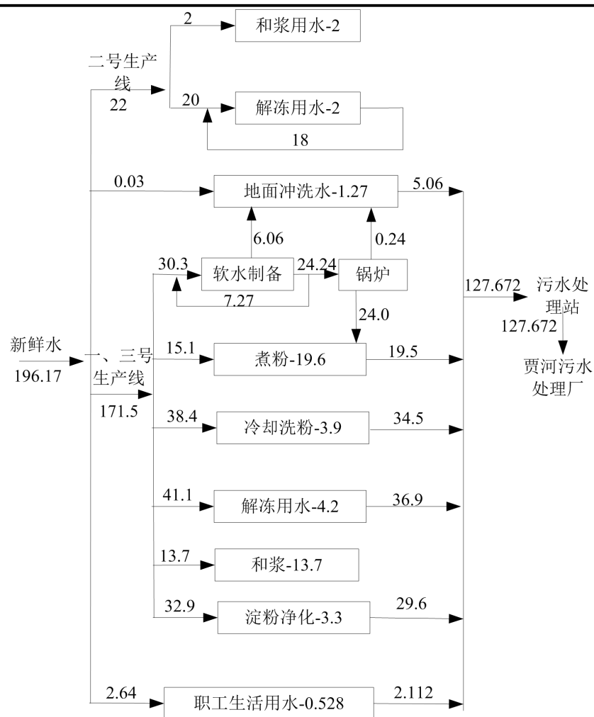
图 2.4 改扩建后全厂给排水平衡图 （单位：m³/d）
