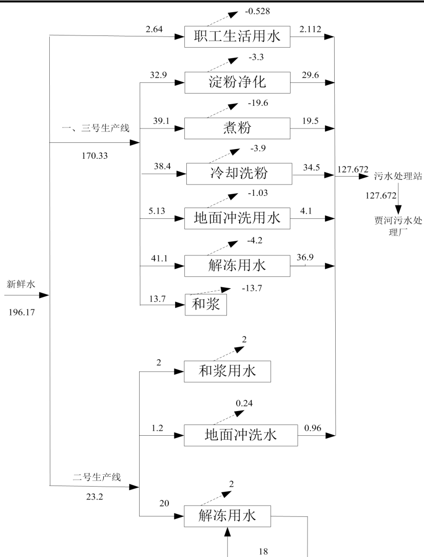
图2-1 现有工程水量平衡图 单位m³/d
