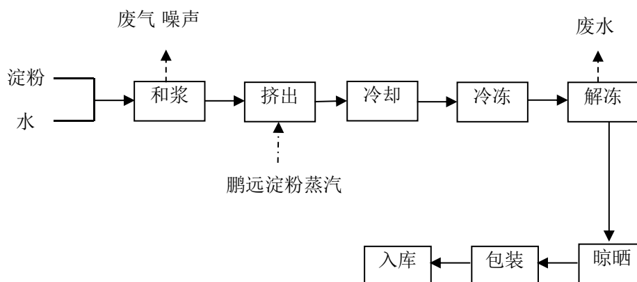
图2-3 现有工程二号生产线工艺流程图
