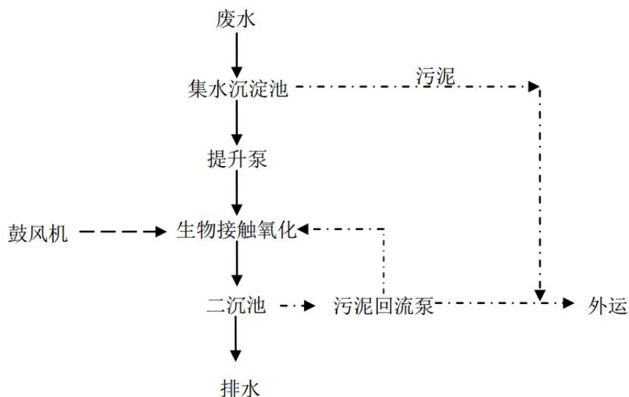
图4-1 厂区污水处理站工艺流程
