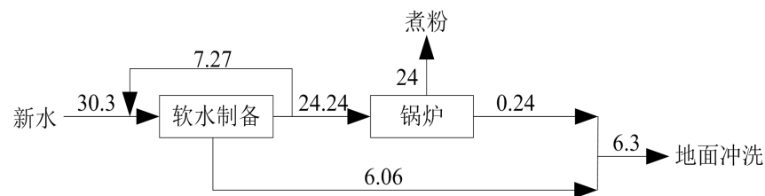
图2-6 扩建项目水量平衡图 单位m 3 /d
