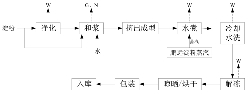
图 2-2 现有工程工艺流程图
