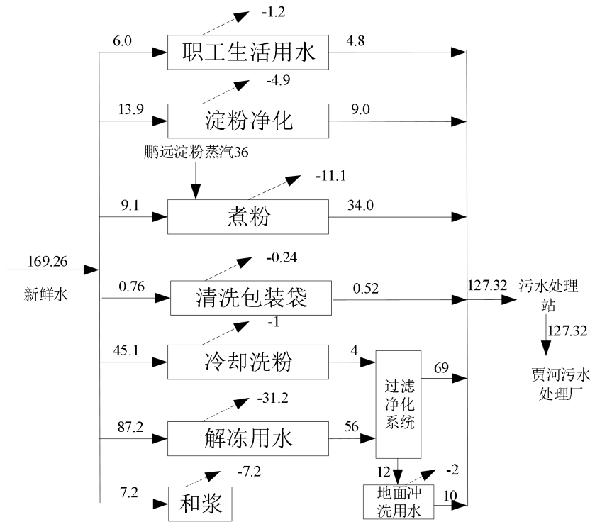
图2-1 现有工程水量平衡图 单位t/d
