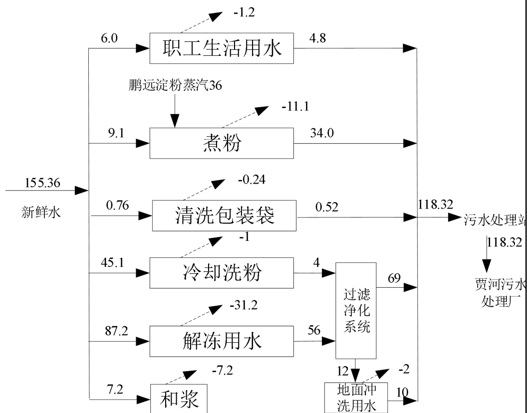
图 2-4 现有工程“以新带老”后水量平衡图 单位 m³/d
