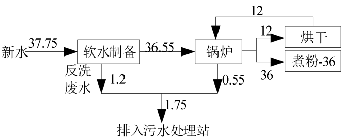
图 2-3 本项目水量平衡图 单位 m 3 /d
