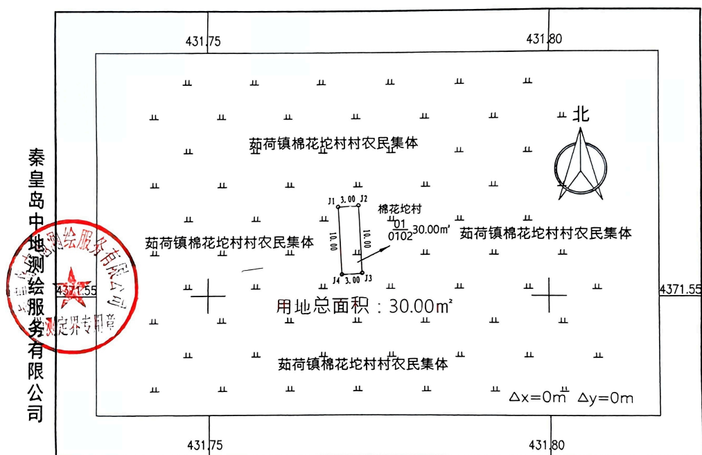
国华投资秦皇岛昌黎500MW海上光伏试点项目地块4建设用地勘测定界图
