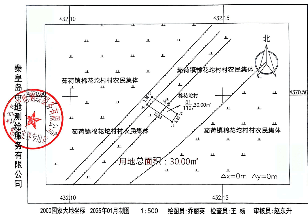
国华投资秦皇岛昌黎500MW海上光伏试点项目地块5建设用地勘测定界图
