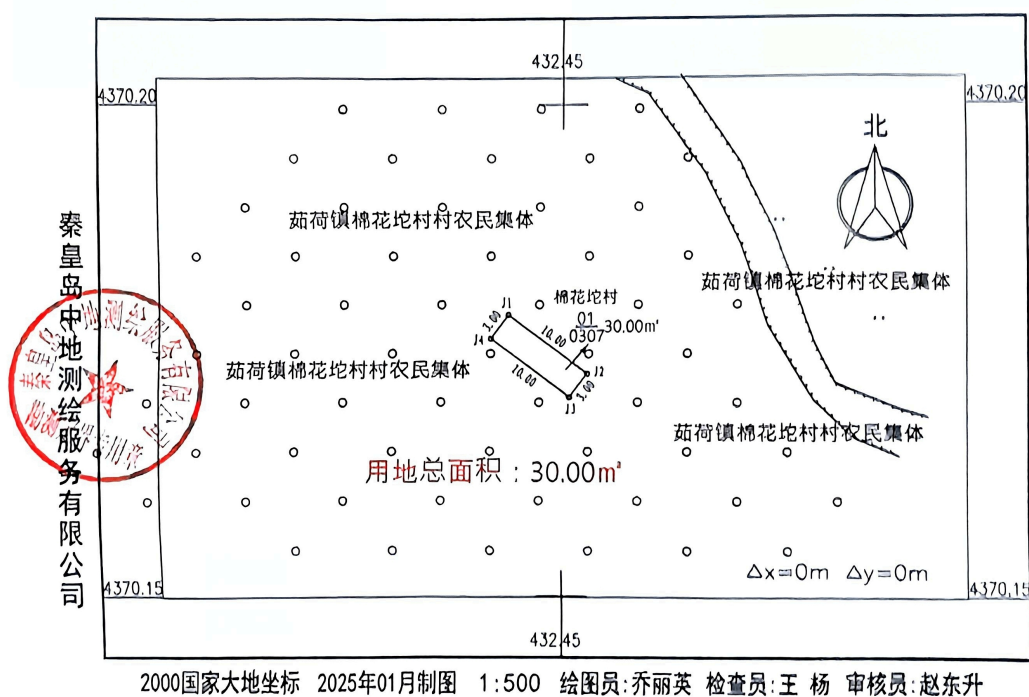
国华投资秦皇岛昌黎500MW海上光伏试点项目地块7建设用地勘测定界图
