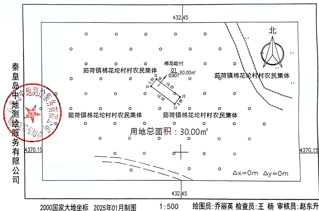
国华投资秦皇岛昌黎500MW海上光伏试点项目地块8建设用地勘测定界图
