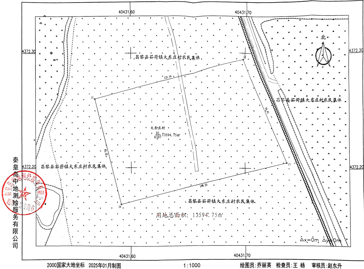
国华投资秦皇岛昌黎500MW海上光伏试点项目升压站建设用地勘测定界图
