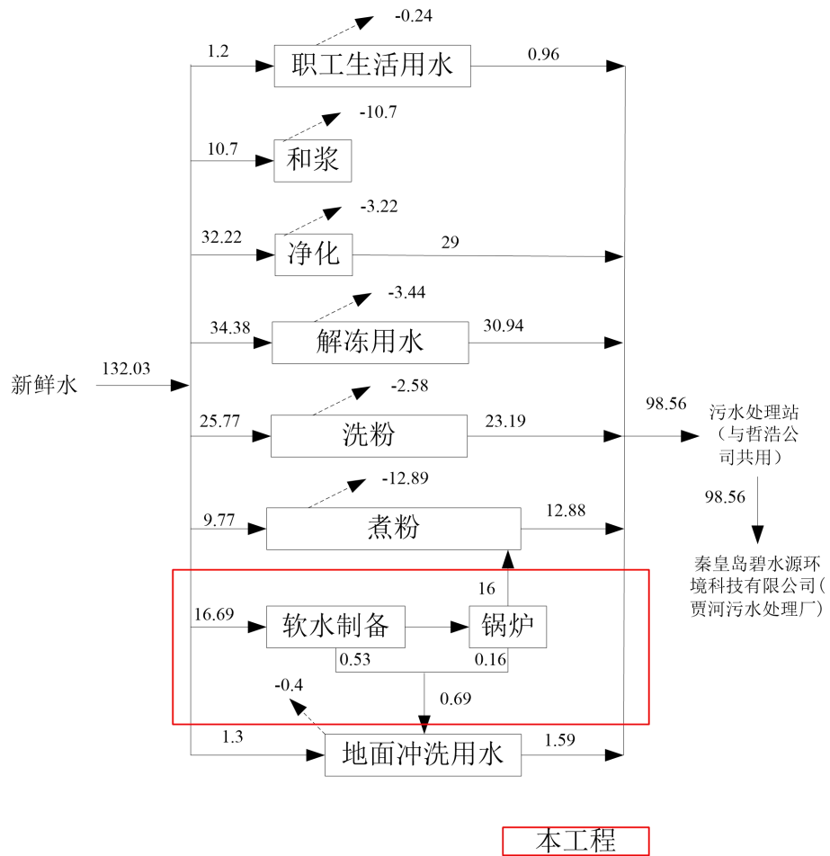
图 2-4 改建完成后全厂水量平衡图 单位 t/d
