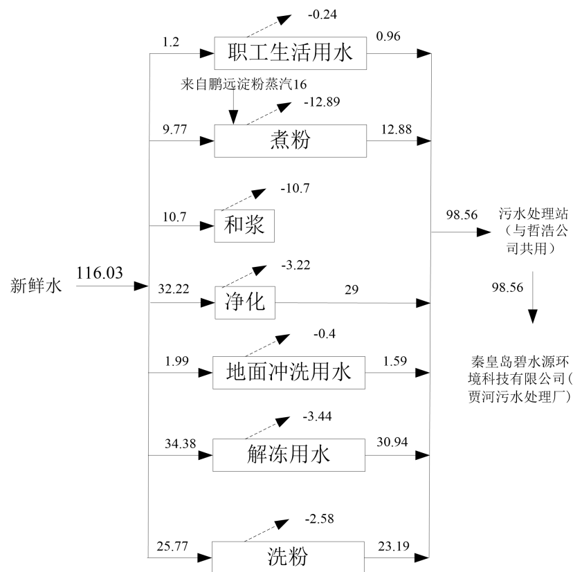
图2-1 现有工程水量平衡图 单位t/d
