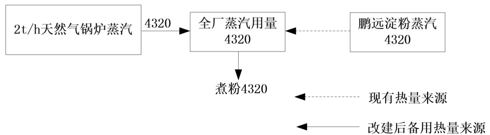
图2-5 全厂蒸汽平衡图 单位t/a
