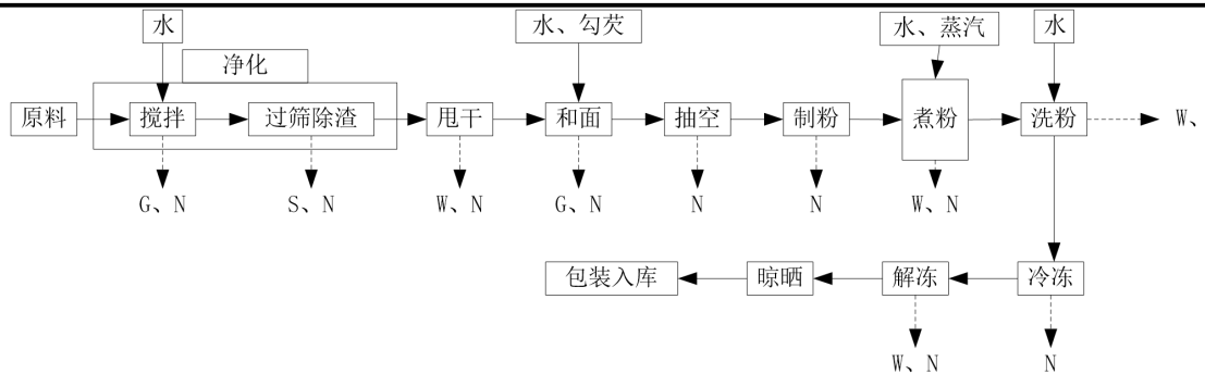
图2-2 现有工程工艺流程图
