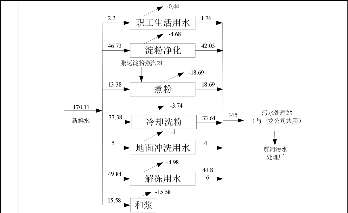
图2-1 现有工程水量平衡图 单位t/d
