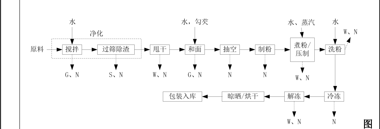
2-2 现有工程工艺流程图
