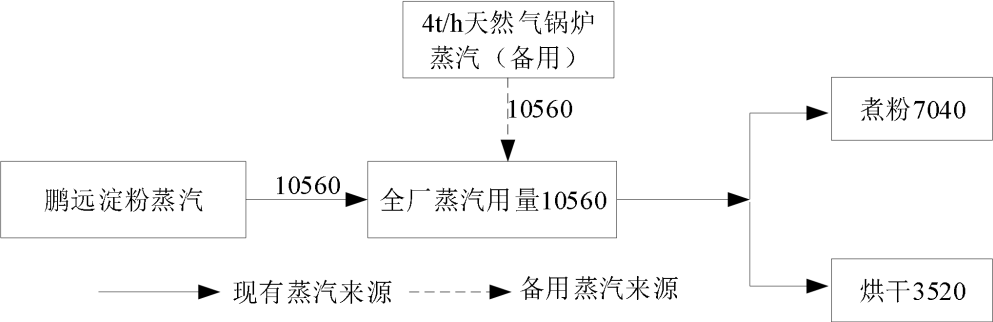
图 2-5 全厂蒸汽平衡图 单位 t/a
