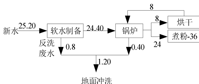
图 2-3 本项目水量平衡图 单位 m³/d
