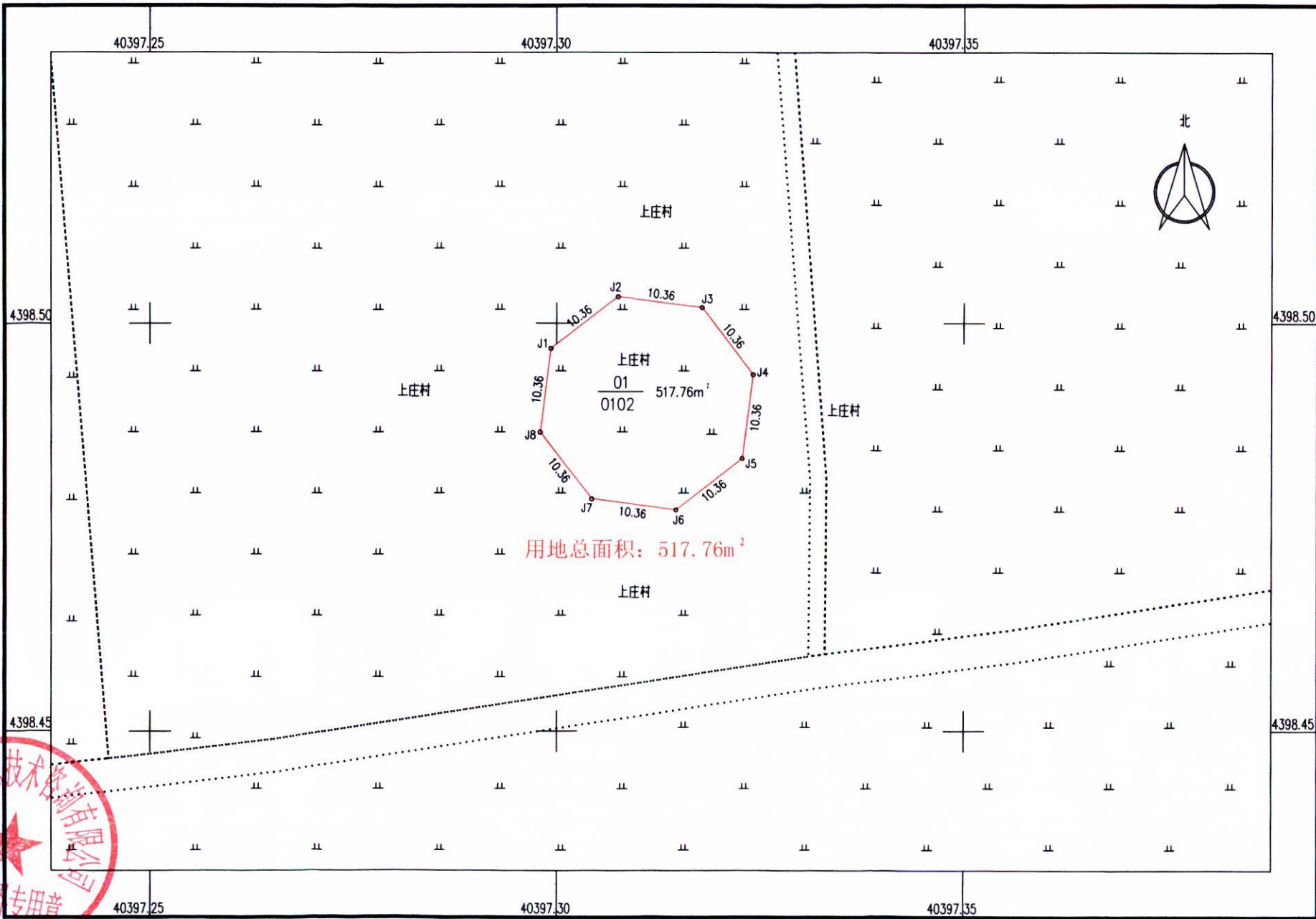
秦皇岛蓝凯新能源有限公司昌黎县朱各庄镇 38.75MW 风力发电项目 (K7号机位) 勘测定界图
