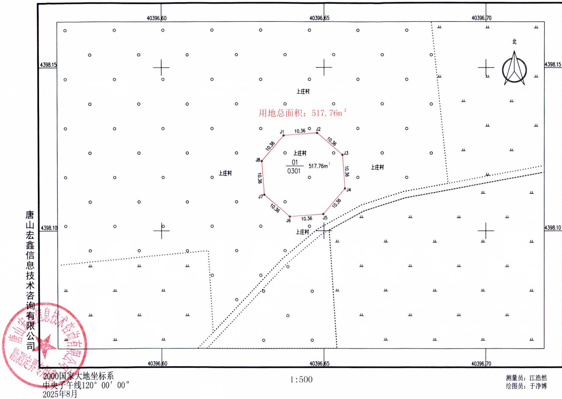
秦皇岛蓝凯新能源有限公司昌黎县朱各庄镇 38.75MW 风力发电项目 (K5号机位) 勘测定界图
