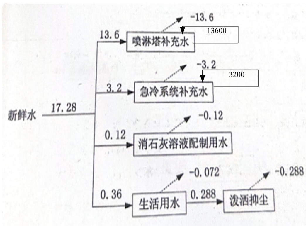
图 2 现有工程水平衡图 单位：m³/d
