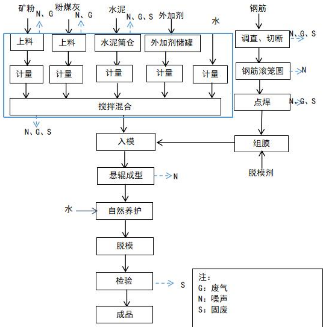
图 2-3 本项目生产工艺流程及产污节点图
